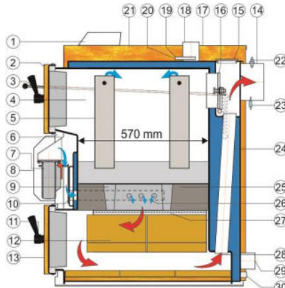
Schéma VIGAS 60,80
