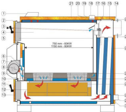
Schéma VIGAS 60,80
