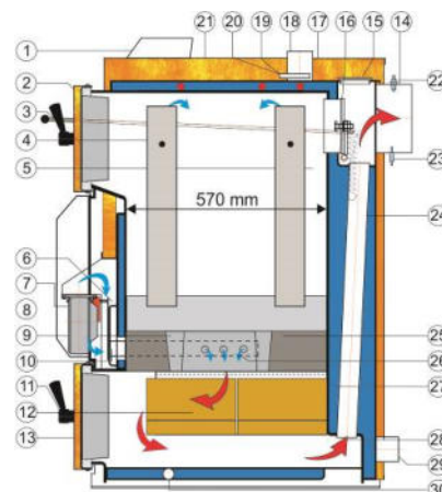
Schéma VIGAS 100
